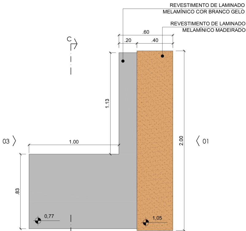
Balcão vista superior sem escala
