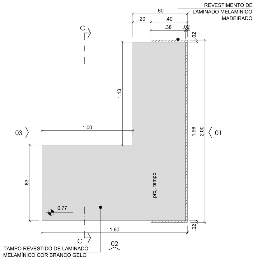
Balcão corte A sem escala
