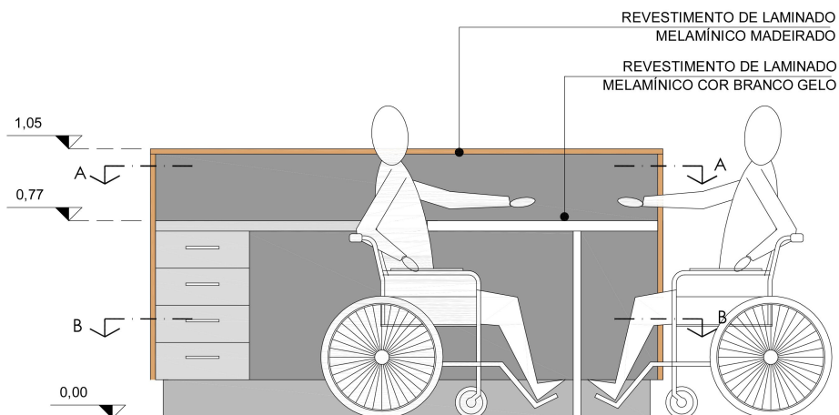
Balcão corte C sem escala
