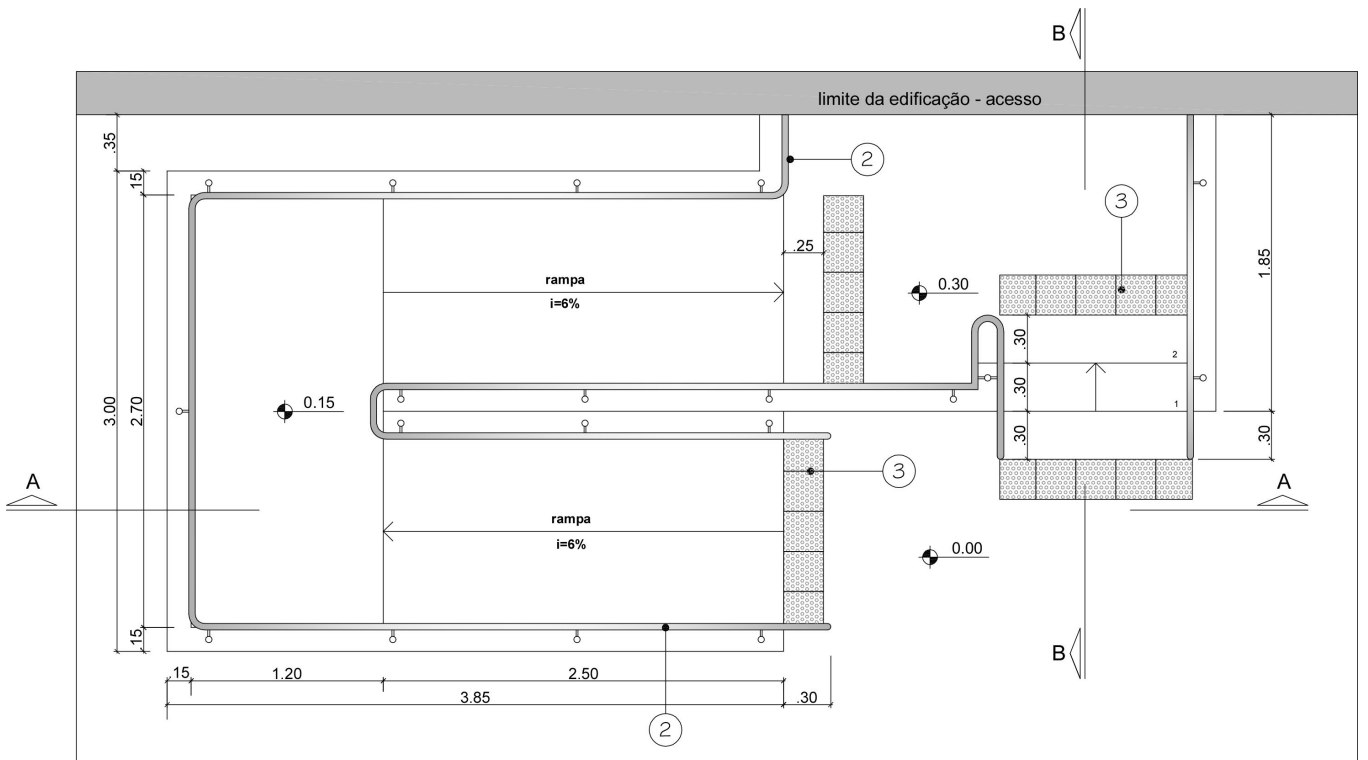
Rampa vista superior sem escala
